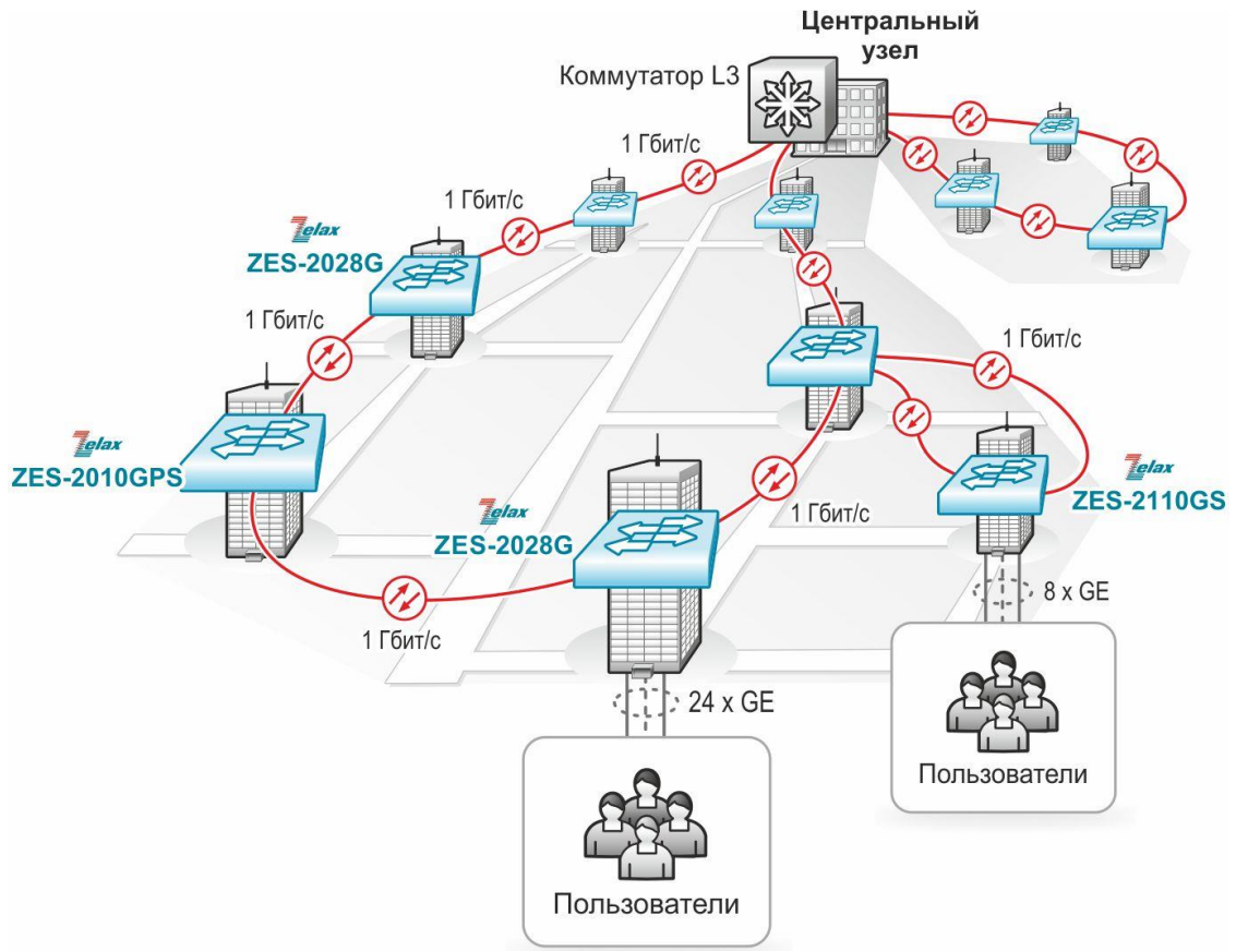
Рис. 1 — Использование коммутаторов ZES-20xxG, ZES-21xxG
