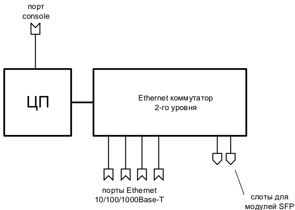
Рис. 3 — Структурная схема коммутаторов ZES-20xxG, ZES-21xxG кроме ZES-2028G(P)S-x-A
