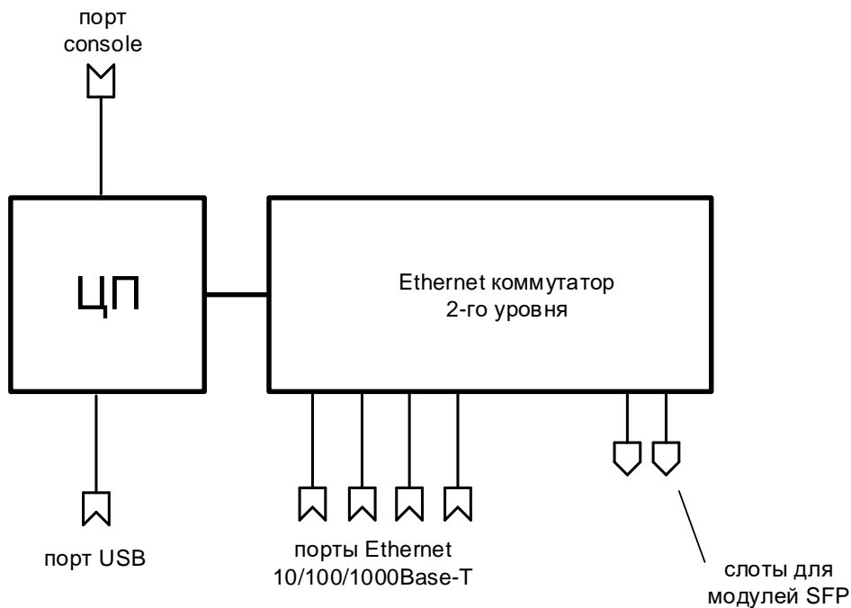
Рис. 2 — Структурная схема коммутаторов ZES-2028G(P)S-x-A
