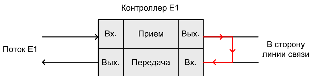
Рис. 2. Шлейф local
