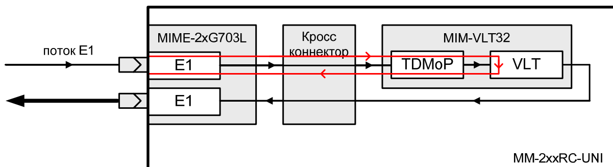
Рис. 4. Шлейф digital
