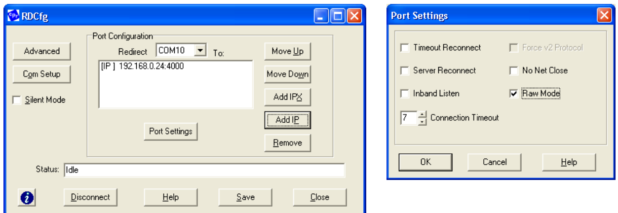
Рис. 12. Настройка программы ComPort Redirector
