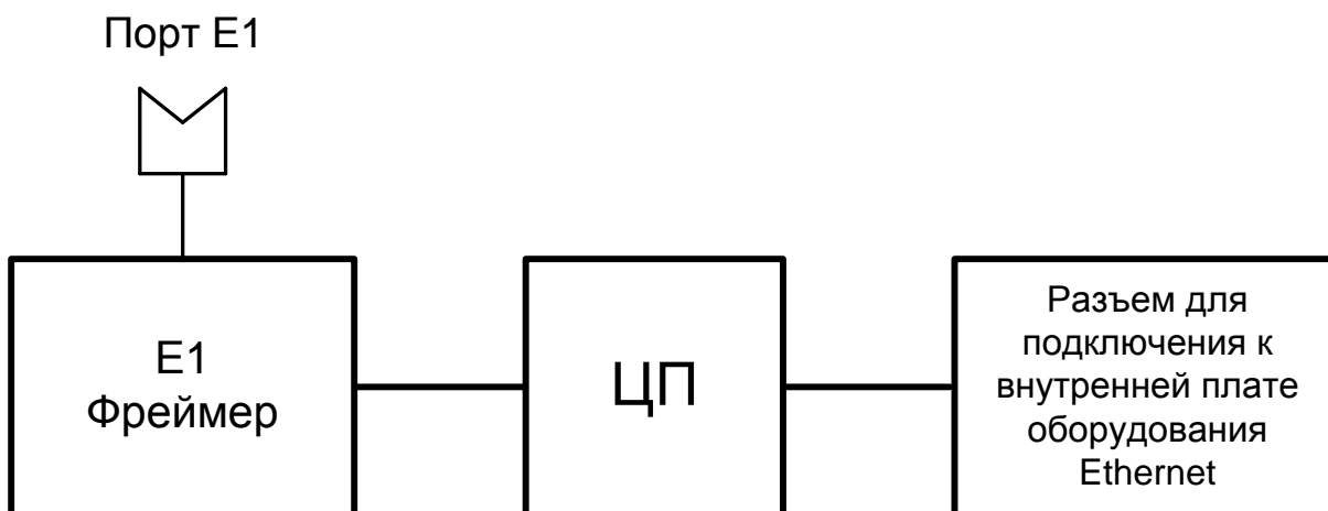
Рис. 9. Структурная схема шлюза MM-101
