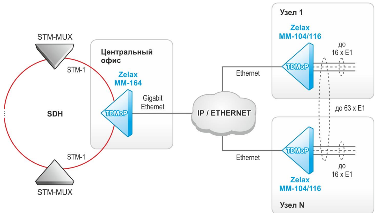
Рис. 5 Выделение/вставка до 126 потоков E1/G.703 из кольцевой сети SDH уровня STM-1 и передача их на оконечные узлы через сеть IP/Ethernet
