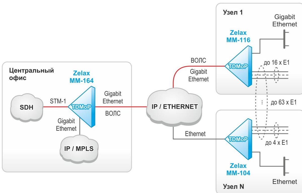
Рис. 4. Агрегация потоков E1, передаваемых через IP/Ethernet-сеть TDMoP-шлюзами MM-104 (MM-116) или MM-132 в поток STM-1
