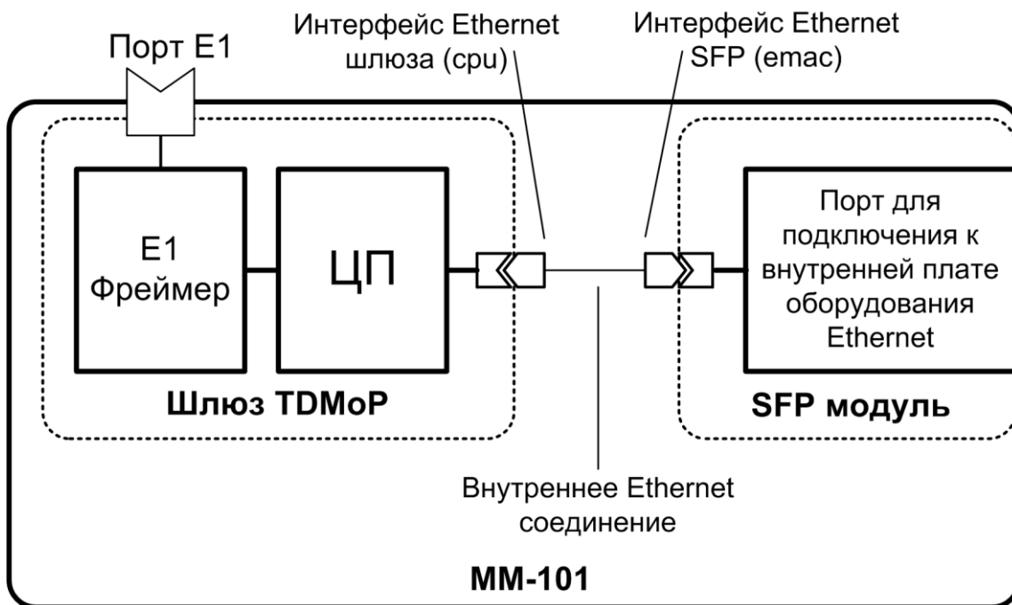
Рис. 10. Логическая схема шлюза MM-101
