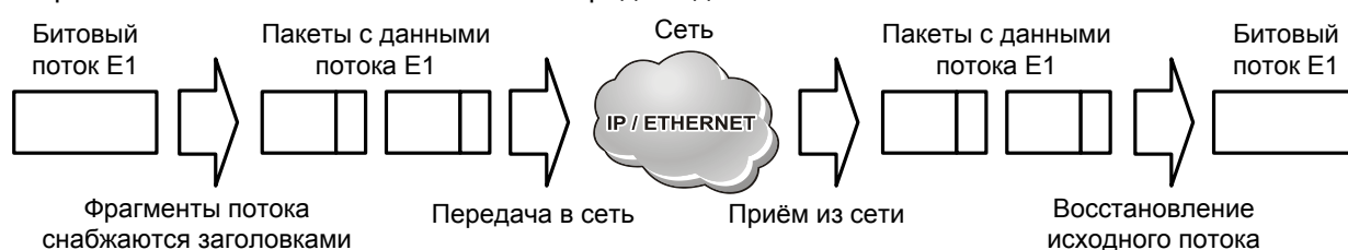
Рис. 6. Схема преобразования потока E1 при его передаче через пакетную сеть
