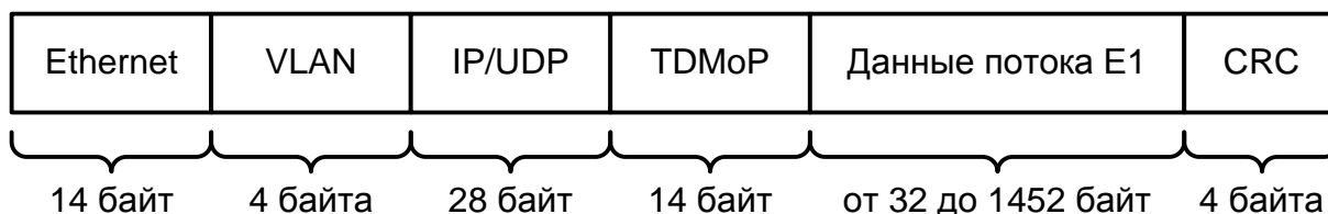
Рис. 7. Формат пакета с данными потока E1
