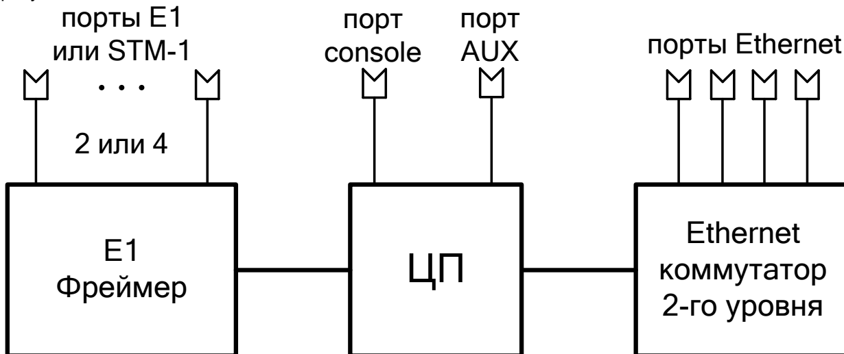
Рис. 8. Структурная схема шлюза MM-104/MM-116/MM-164
