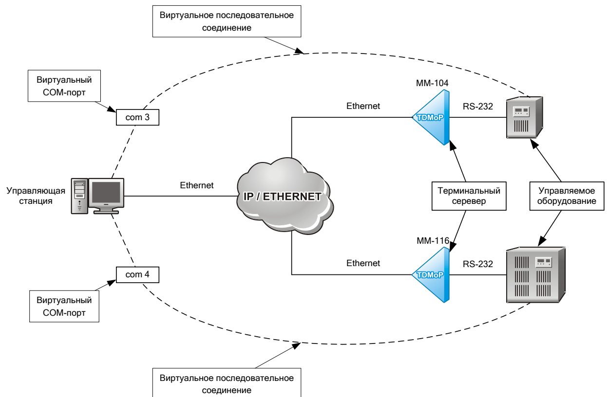
Рис. 11. Схема организации удаленного управления оборудованием по интерфейсу RS-232 через пакетную сеть при помощи встроенного терминального сервера
