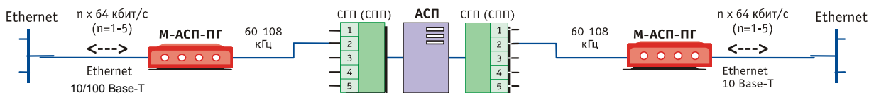
Рис. 3. Пример объединения сетей Ethernet 10/100 Base-T с помощью модема М-АСП-ПГ
