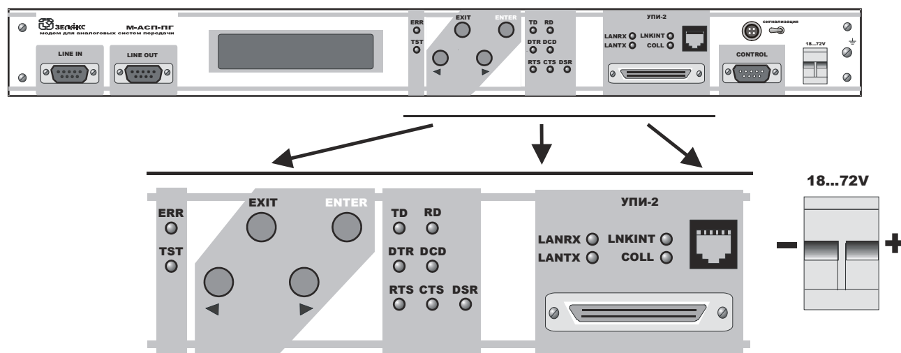
Рис. 7. Передняя панель модема М-АСП-ПГ
