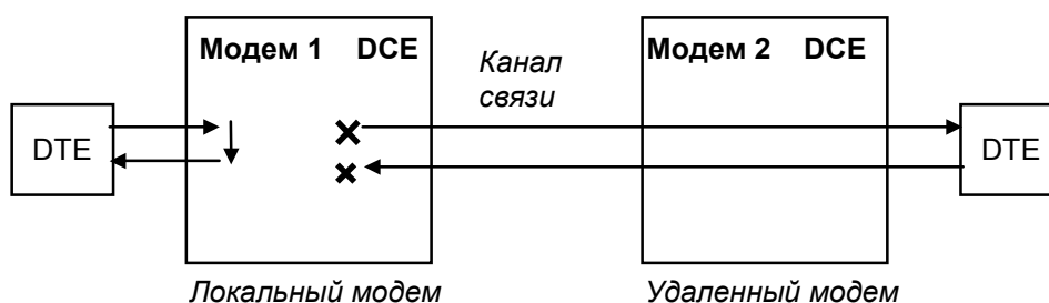
Рис. 19. Проверка в режиме LL - «местный цифровой шлейф»
