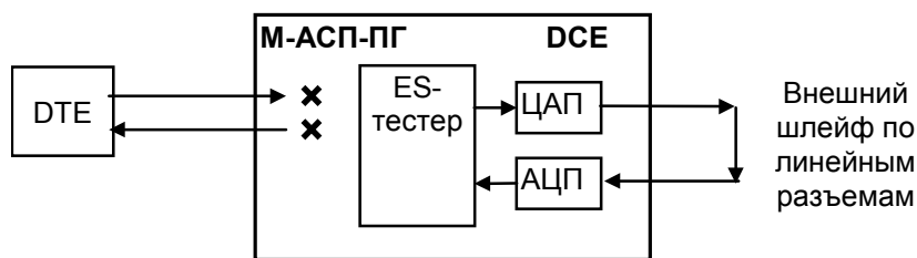
Рис. 14. Проверка в режиме AL-ES - «Аналоговый шлейф» с использованием ES-тестера
