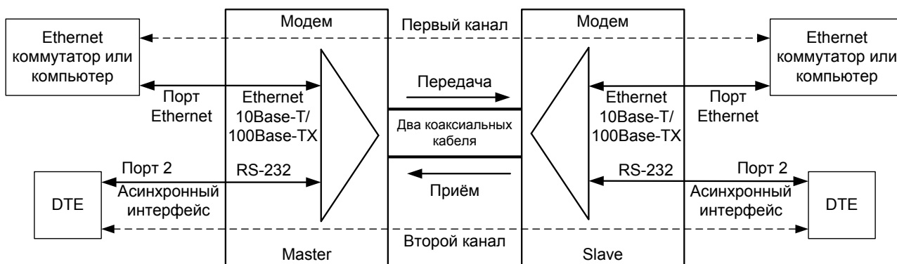
Рис. 3. Структура каналов связи с использованием модемов М-30Ш; линия выполнена на основе двух коаксиальных кабелей
