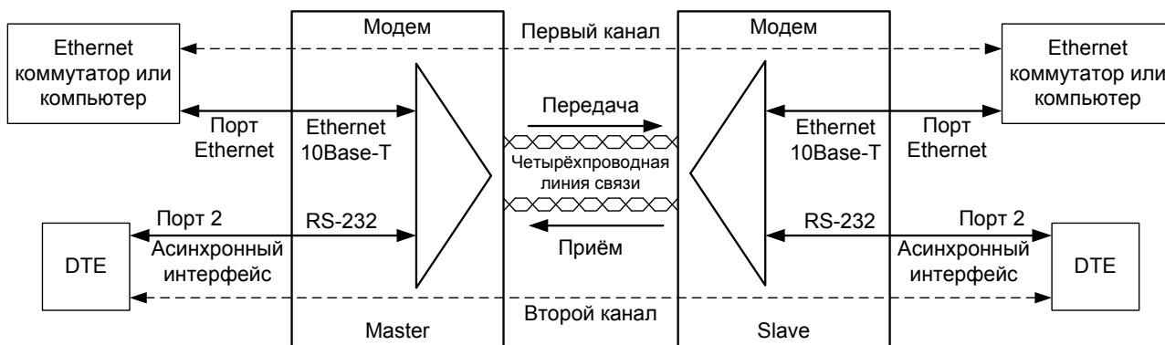
Рис. 1. Структура каналов связи с использованием модемов М-30А
