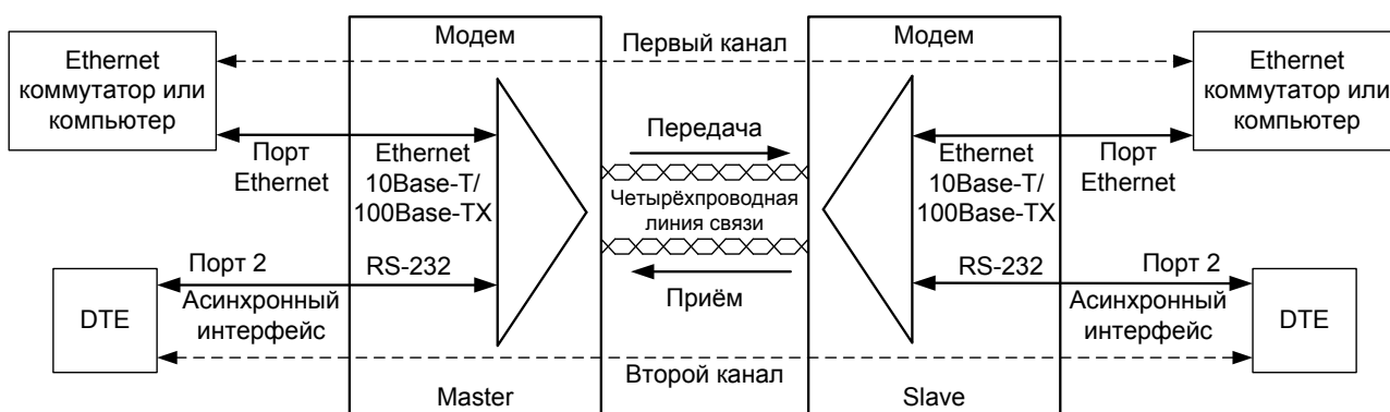
Рис. 2. Структура каналов связи с использованием модемов М-30Б или М-30Ш
