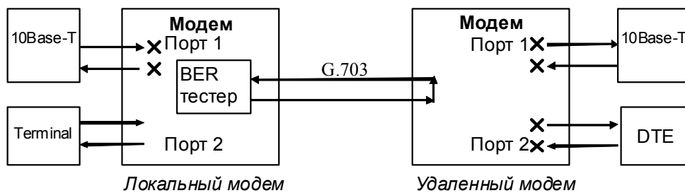
Рис.8. Проверка канала G.703
