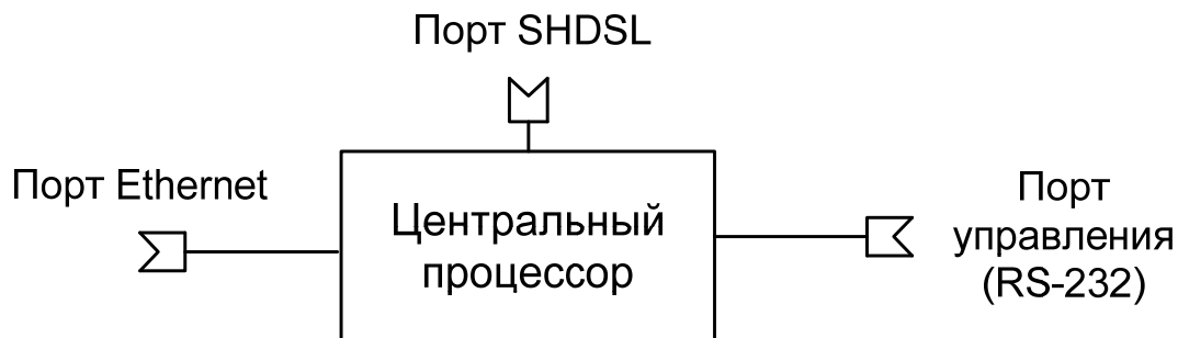
Рис. 2. Структурная схема модема
