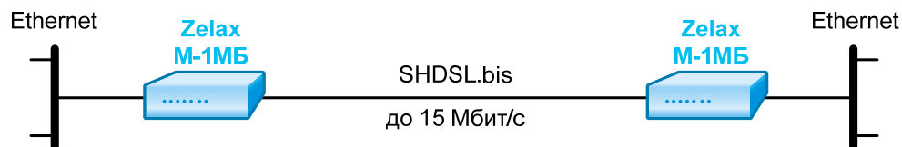
Рис. 1. Передача данных Ethernet по одной медной витой паре на скорости до 15296 кбит/с
