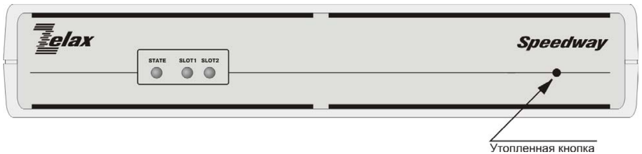
Рис. 16. Вид передней панели изделий MM-2xx настольного исполнения
