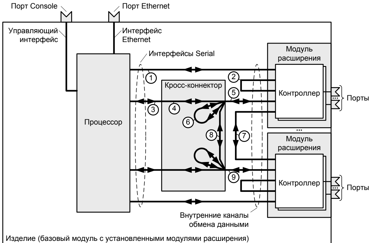
Рис. 5. Структурная схема изделий MM-201RC-UNI, MM-202RC-UNI, MM-211RC-UNI, MM-212RC-UNI и MM-502RC-UNI
