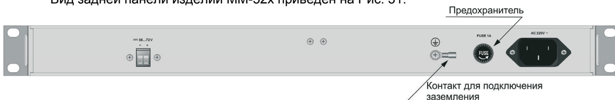
Рис. 31. Вид задней панели изделия MM-52x
