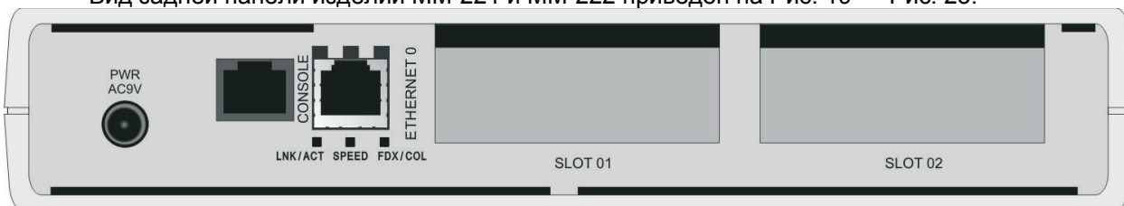
Рис. 21. Вид задней панели изделий MM-221x-AC9 и MM-222x-AC9 настольного исполнения с питанием от сети переменного тока
