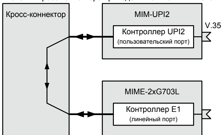
Рис. 4. Передача данных V.35 через канал E1
