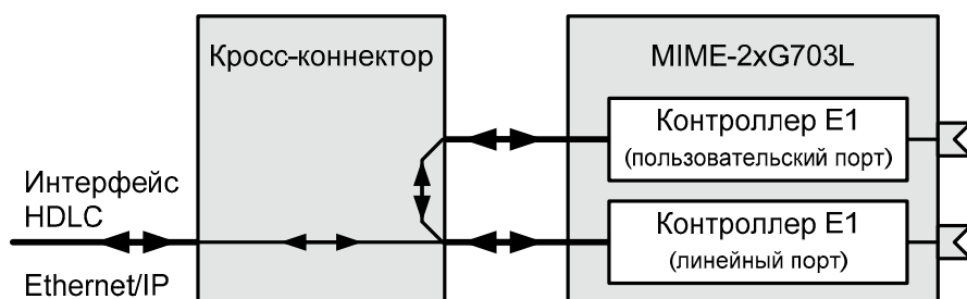
Рис. 7. Передача данных Ethernet/IP через выбранные таймслоты потока E1 в режиме извлечения — вставки
