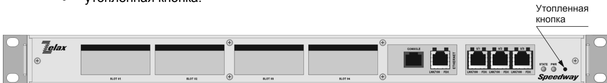
Рис. 20. Вид передней панели изделий MM-525RC-UNI
