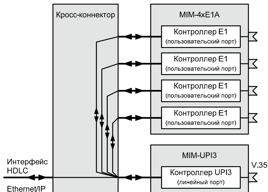
Рис. 10. Передача данных Ethernet/IP и четырёх потоков E1 через канал V.35
