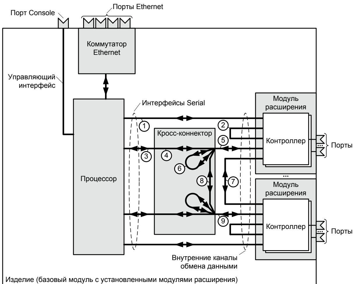
Рис. 3 Структурная схема изделия ММ-225, ММ-525
