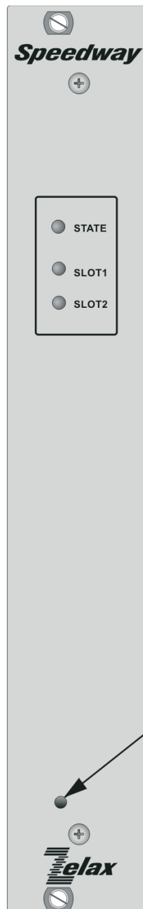
Рис. 17. Вид передней панели изделий ММ-22х для установки в конструктив Р-510
