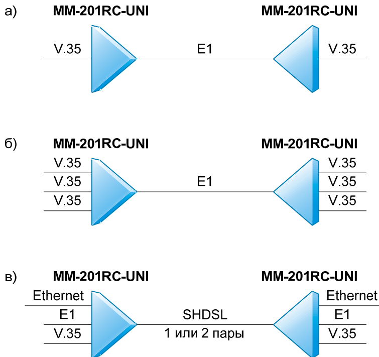
Рис. 1. Примеры использования модуля совместно с устройствами MM-20x
