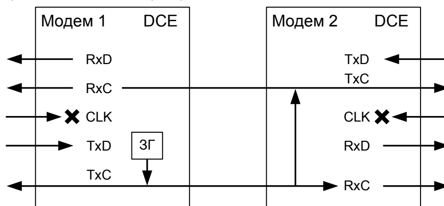
Рис. 19. Синхронизация в режиме Receiver модема 2 (модем 1 — синхронизация Internal).
