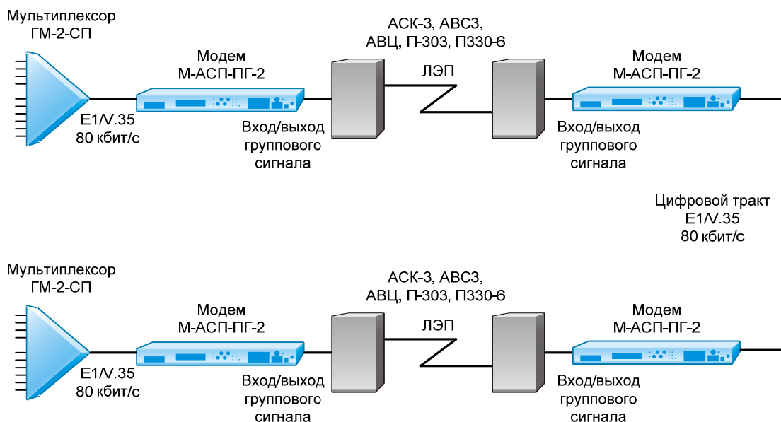
Рис. 2. Организация цифрового канала 80 кбит/с в тракте АСП по ЛЭП с использованием цифрового транзита.
