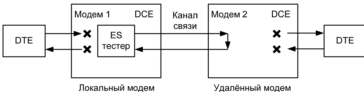
Рис. 10. Проверка в режиме RDL-ES — «удаленный шлейф» с использованием ES-тестера
