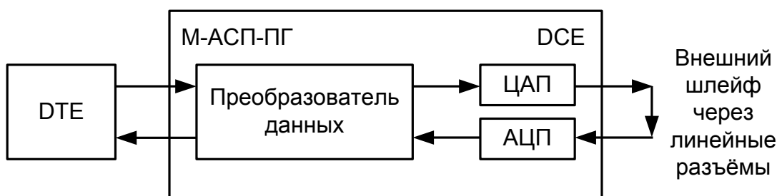
Рис. 14. Проверка в режиме AL — “Аналоговый шлейф”
