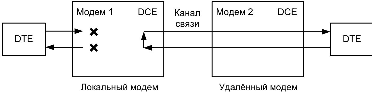
Рис. 15. Проверка в режиме DL — “цифровой шлейф”
