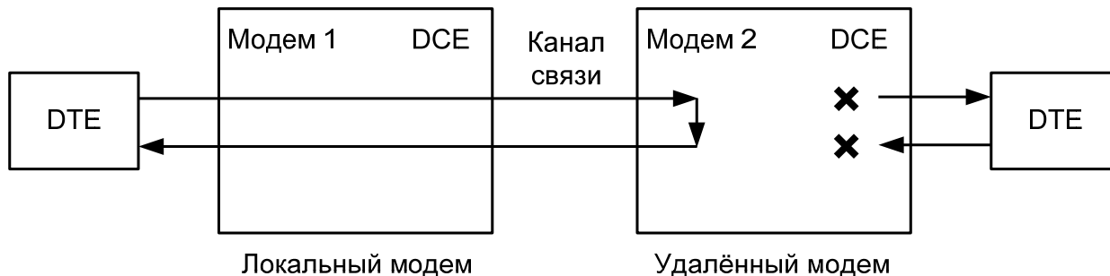
Рис. 13. Проверка в режиме RDL “удаленный цифровой шлейф”.
