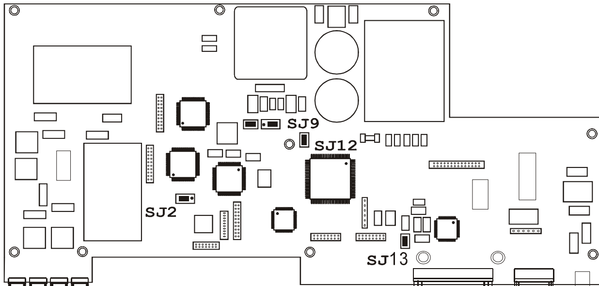
Рис. 5. Расположение элементов на плате модема М-АСП-ПГ
