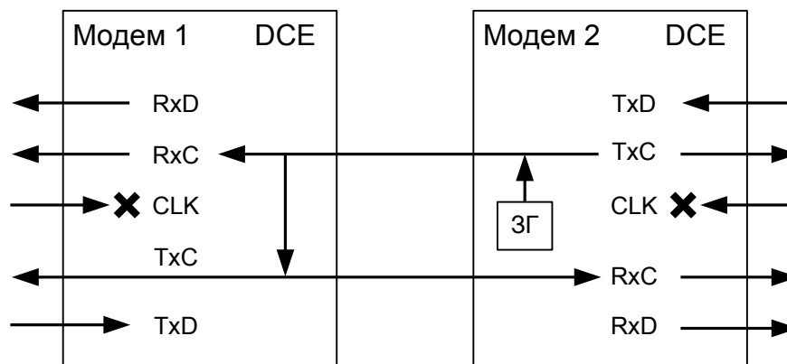
Рис. 23. Синхронизация в режиме Internal модема 2 (модем 1 — синхронизация Receiver).
