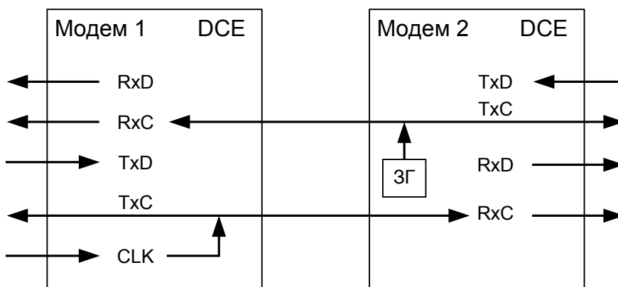
Рис. 20. Синхронизация в режиме Internal модема 2 (модем 1 — синхронизация External).
