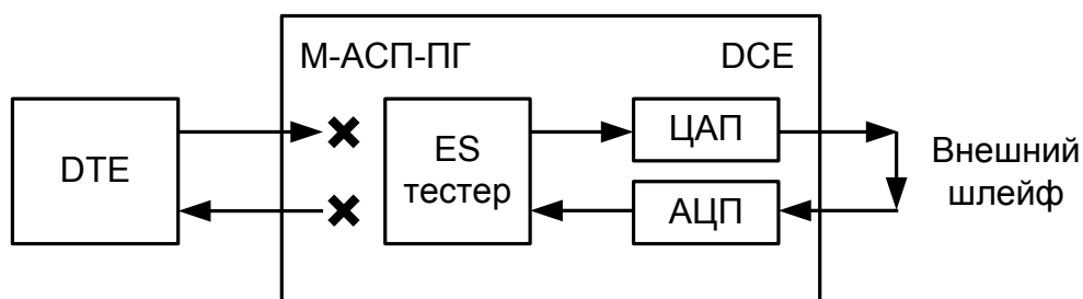
Рис. 12. Проверка в режиме подключения ES-тестера к каналу связи
