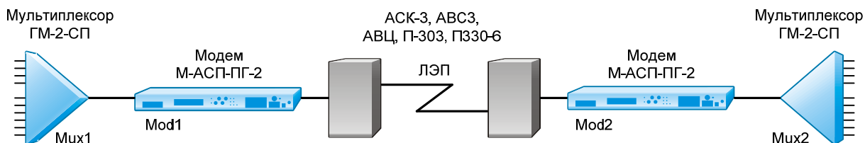
Рис. 25. Организация связи между мультиплексорами через модемы М-АСП-ПГ-ЛЭП
