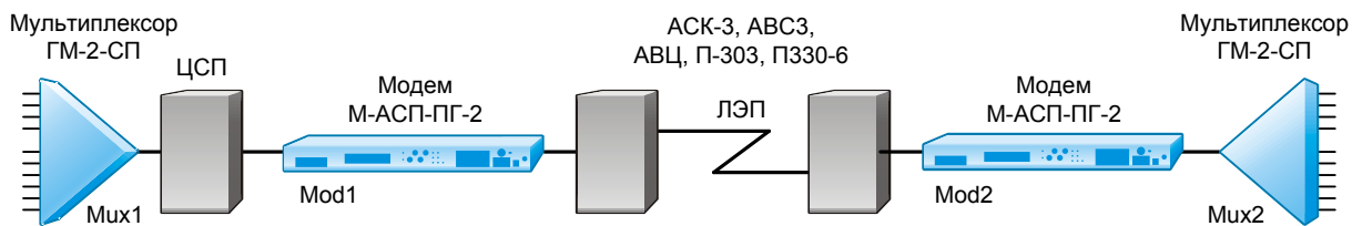
Рис. 26. Организация связи между мультиплексором и модемом через ЦСП
