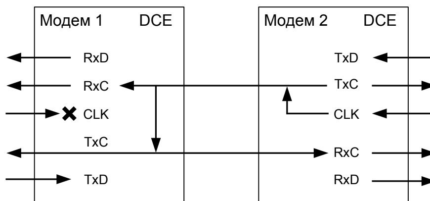
Рис. 24. Синхронизация в режиме External модема 2 (модем 1 — синхронизация Receiver).
