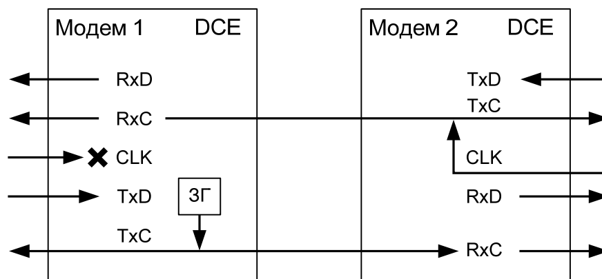
Рис. 18. Синхронизация в режиме External модема 2 (модем 1 — синхронизация Internal)
