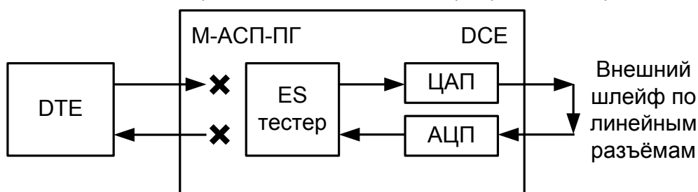
Рис. 11. Проверка в режиме AL-ES - «Аналоговый шлейф» с использованием ES-тестера
