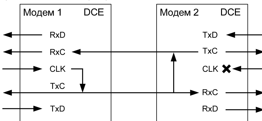
Рис. 22. Синхронизация в режиме Receiver модема 2 (модем 1 — синхронизация External).
