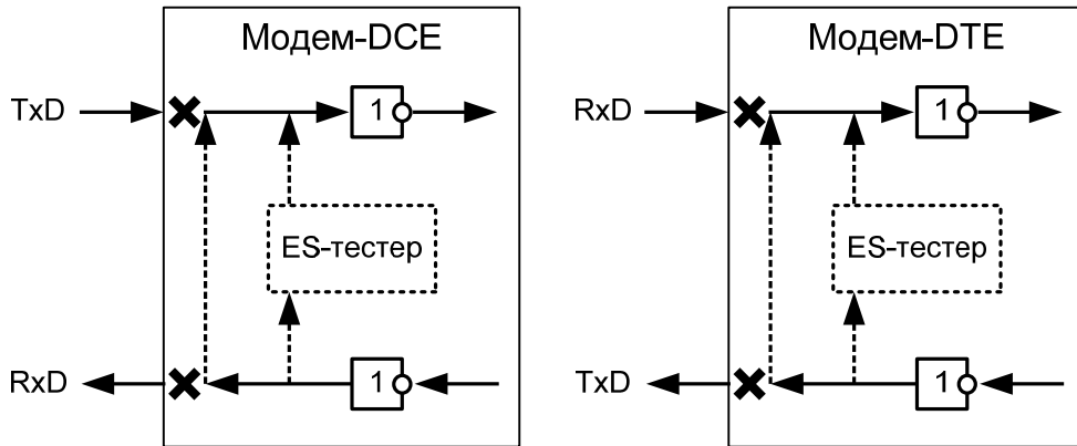
Рис.28. Включение инверторов для цепей RxD и TxD в тестовых режимах RDL/AL-ES, DL .
