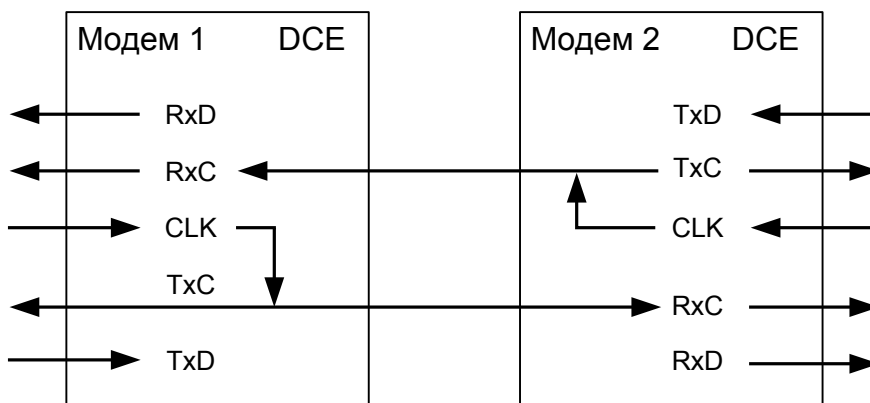
Рис. 21. Синхронизация в режиме External модема 2 (модем 1 — синхронизация External).
