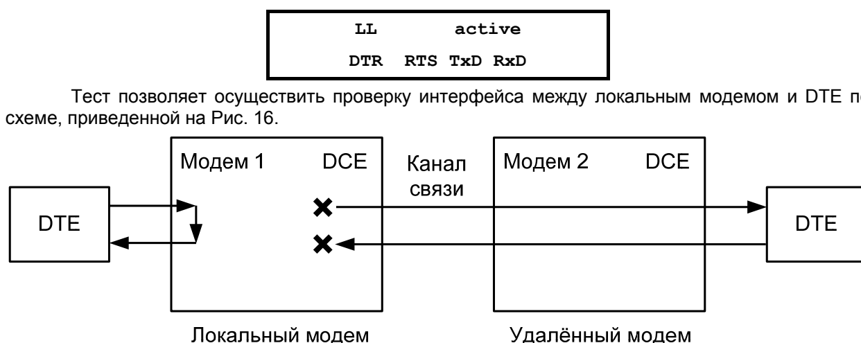
Рис. 16. Проверка в режиме LL — “местный цифровой шлейф”
