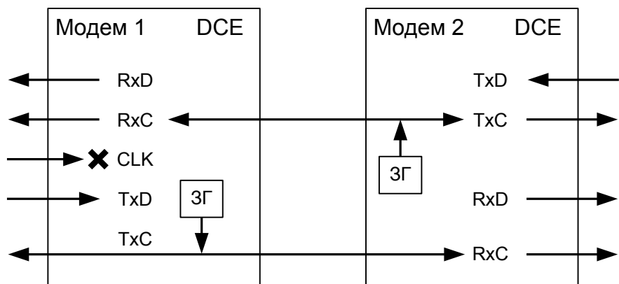
Рис. 17. Синхронизация в режиме Internal модема 2 (модем 1 — синхронизация Internal)
