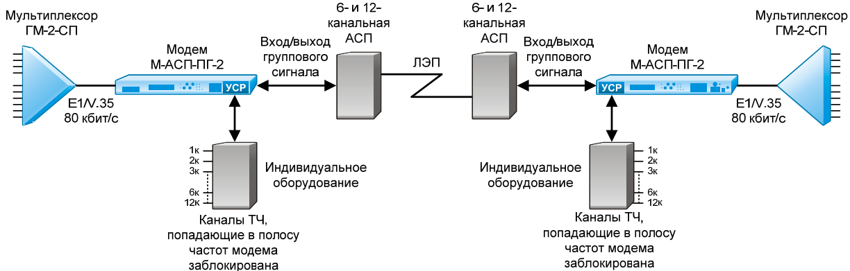
Рис. 3. Включение модемов М-АСП-ПГ-2 вер. ЛЭП в групповой тракт 6-ти и 12-канальных систем с сохранением передачи незанятых модемом каналов ТЧ
