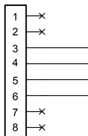
Вилка RJ-45
