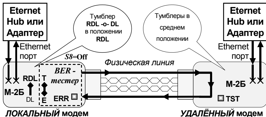
Рис. 12 BER-тестер в режиме RDL
